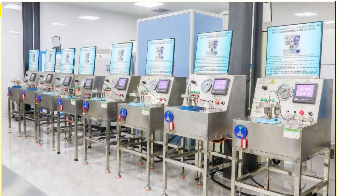
Batterie d'appareils de test de durée de vie de trains thermostatiques. Chaque appareil est équipé d'un enregistreur de paramètres et de nombre de cycles. (Laboratoire Ultimheat).
